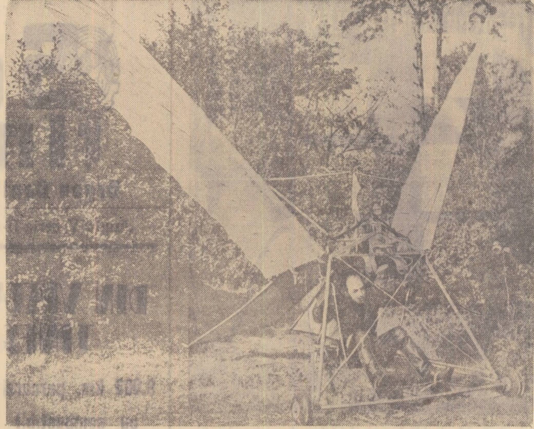
Un avion sovietic a construit un nou tip de aparat de zbor. Experimentele făcute cu acest aparat de zbor cu aripi ornitoptere au arătat că cele două aripi ușoare care sînt puse în mișcare de un motor de 3 CP desfișoară o forță de 21 kg. După calculele teoretice acest aparat poate purta un om în vîzduh cu o viteză pînă la 100 km pe oră. Foto: TASS
