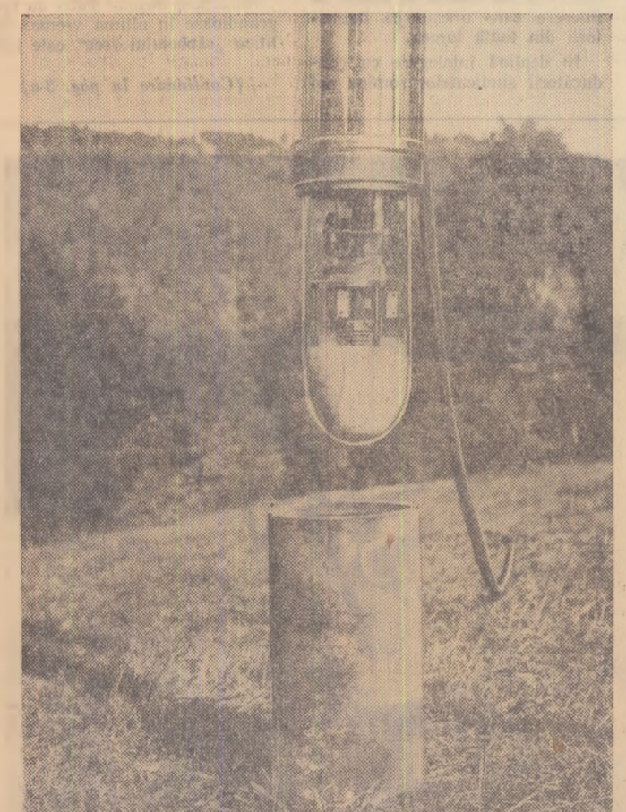
Inginerul Michal Krajcik din Bratislava a instalat un aparat cilindric de televiziune într-o sondă geologică și a obținut prin intermediul lui informații asupra straturilor de piatră. Aparatul de televiziune poate fi aflat pînă la o adîncime de 250 metri și se prevede că după unele adaptări speciale el va putea ajunge pînă la o adîncime de 1.500 metri. În foto: fixarea camerei de televiziune într-o sondă geologică. Foto: C.T.K.
