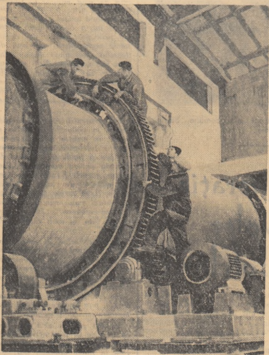
Pe șantierul combinatului de Ingrășăminte azotoase de la Rosnov, regiunea Bacău, lucrările de construcții și montaj sînt în toi. Iată în fotografie echipa de montori condusă de Constantin Barossi efectuînd montarea tamburilor de răcire.
