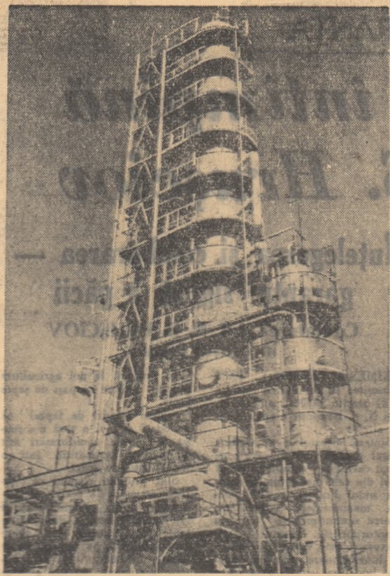
În fotografie: rafinăria nr. 10 Onești, instalația de fracționare gaze.
