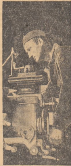
Muncitorul fruntaș Gheorghe Rusu de la Uzinele „Iosif Ranghet” din Arad controlând coaxialitatea unuia din strungurile produse de întreprindere.
