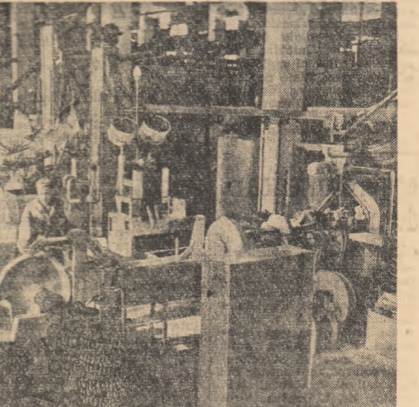
La Uzina „Seltzhozapeti” din Krasnodar a început verificarea primului sector al secției automate pentru producerea lanțurilor cu role pentru combinele autopropulșate. Aici s-au instalat șapte linii automate. Secția este deservită de numai șase oameni. Foto: TASS-Moscova
