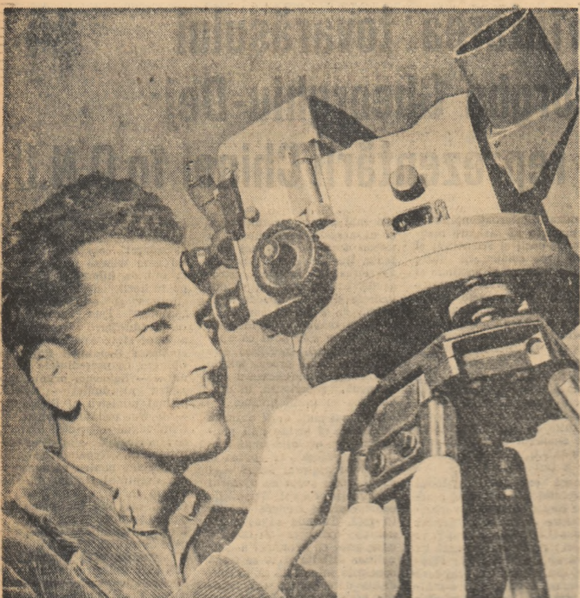
Urmărirea balonului pilot cu teodolitul aerologic pentru măsurarea direcției și vitezei vântului în atmosfera înaltă la Stația meteorologică din Cluj. Foto: A. VIERU
