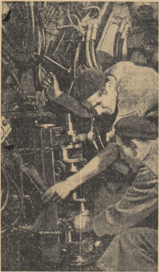
Ultima verificare. Operațiile corespund întocmai schiței tehnice. Maistrul Gheorghe Căldăre împreună cu Chițu Ioan, verifică operațiunile de uzinare executate cu noua mașină agregată pentru găurirea arborelui cotii, mașină concepută și realizată de către colectivul de ingineri și tehnicieni al Uzinelor de tractoare „Ernst Thälmann” din Orașul Stalin.
