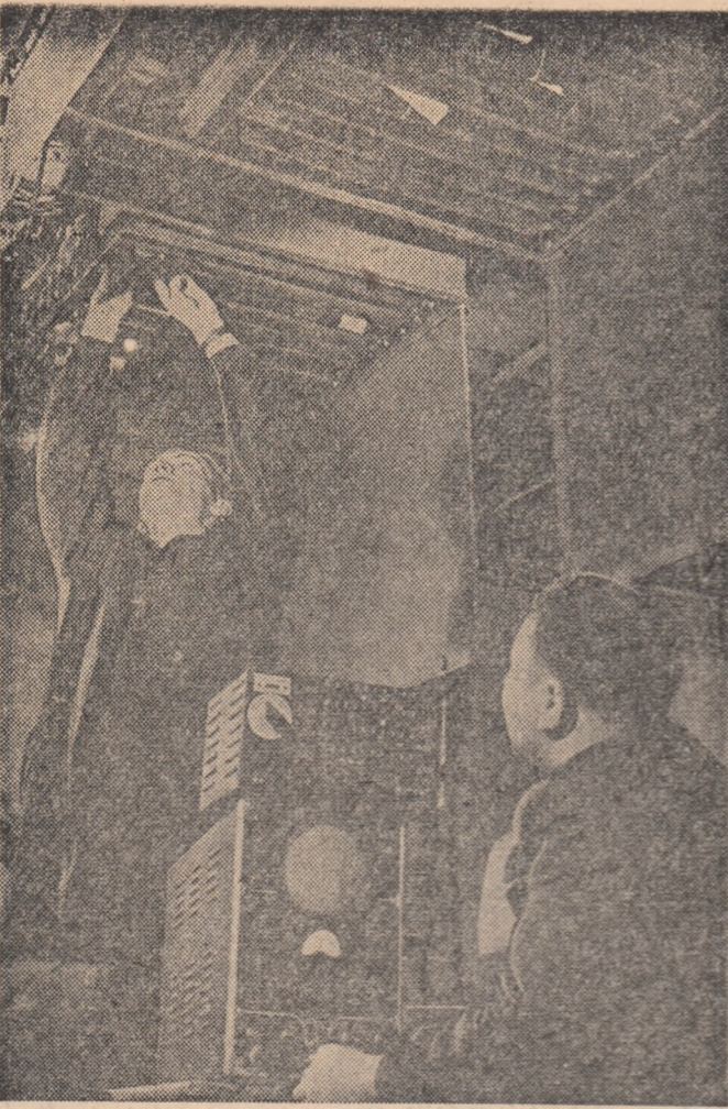
În apropiere de orașul Alma-Ata, capitala R.S.S. Kazah, la 3333 metri deasupra nivelului mării, se construiește stațiunea științifică pentru studierea particulelor cosmice. În foto: montarea aparatului științific.
