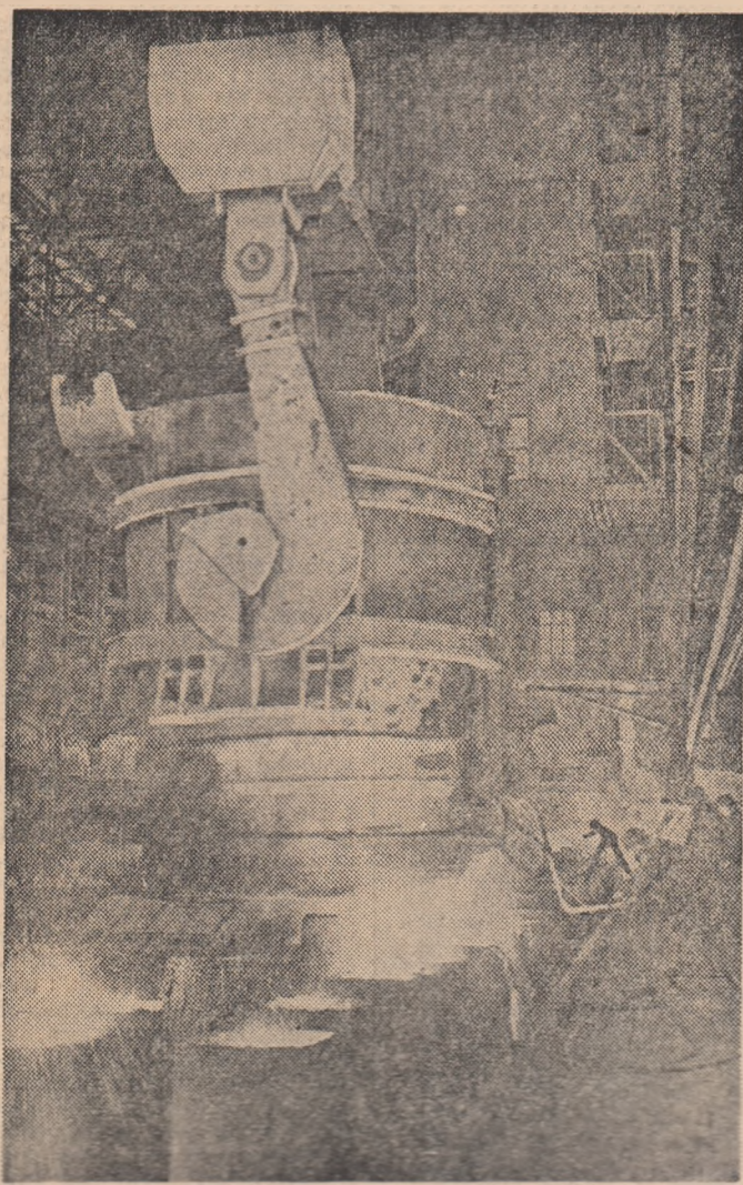
Un moment important: la oțelăria Siemens-Martin din Hunedoara o nouă țară se toarnă în linghiere.
