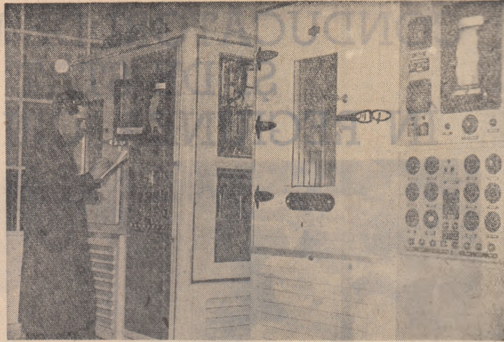
Țara noastră exportă astăzi produse electronice în multe țări ale lumii. V-ați gândit vreodată cum reacționează aceste produse în condițiile climatice ale unor țări îndepărtate? Este într-o sală a camerelor climatice pentru studii comparativă produselor electrotehnice în condiții variate de umiditate, presiune, temperatură.
