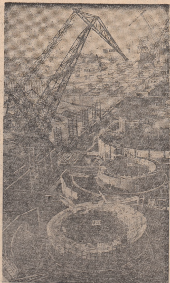
Pe pantionul hidrocentralei de la Votkinsk, U.R.S.S. În cursul acestui an va fi zăgăzuită albia fluviului Kama și vor intra în funcție primele hidroagregate. Aspect de pe pantion
