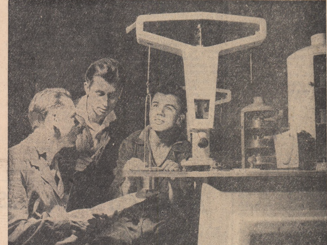
De curînd întreprinderea „Tehnometal” din Capitală a executat un nou prototip de aparat necesar determinării umidității textilelor. Țăstori Atanasie Nodolea, Gh. Suditu și Dumitru Duha, verifică asamblarea perfectă a balantei de la unul dintre noile aparate.
