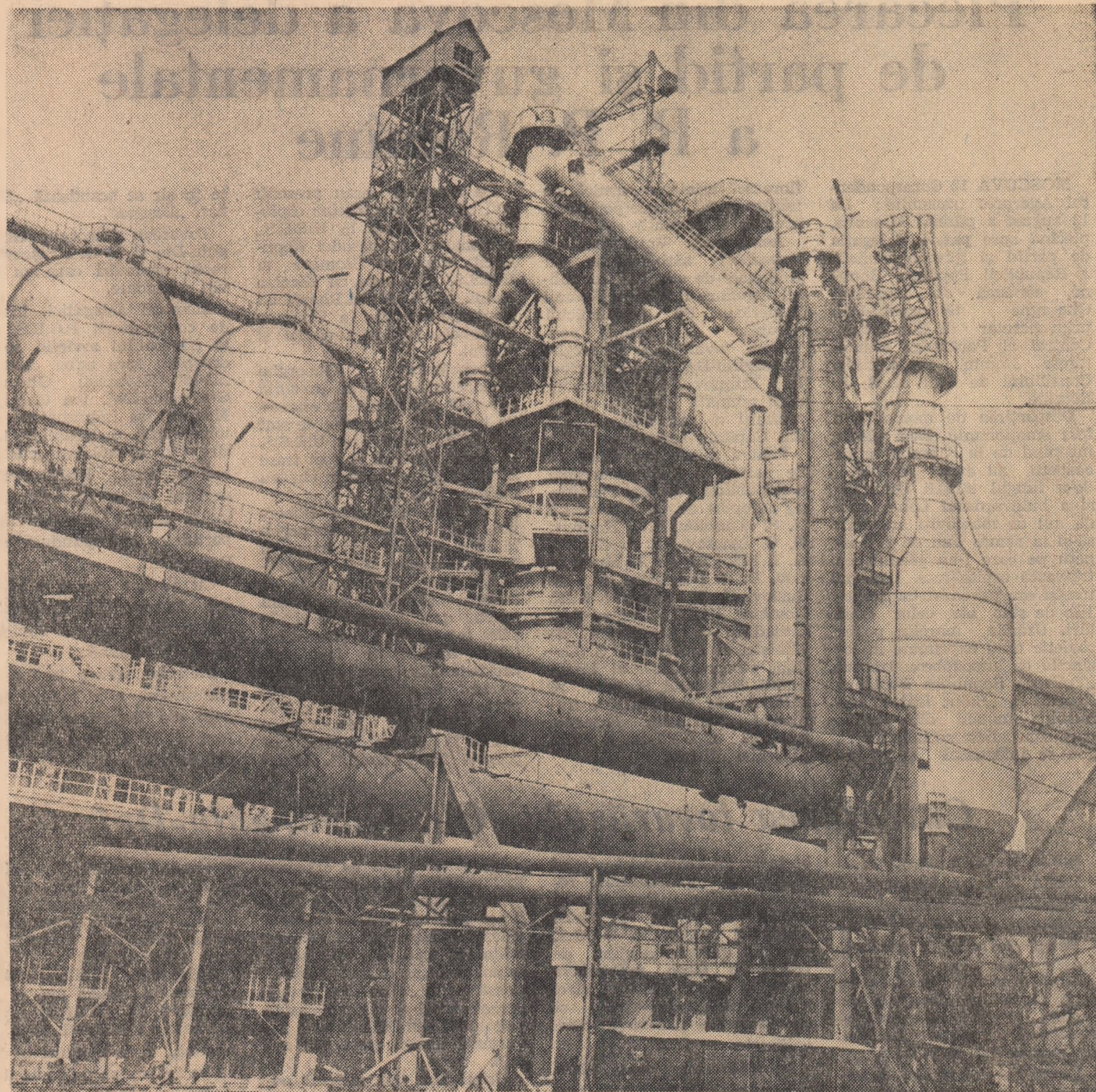
Noul furnal de 700 m.c. intrat recent în funcțiune
