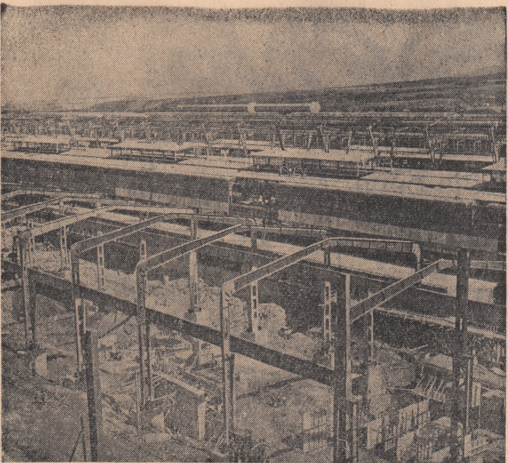
Vedere de ansamblu a laminorului de profile mici și mijlocii care se află în construcție la Hunedoara
