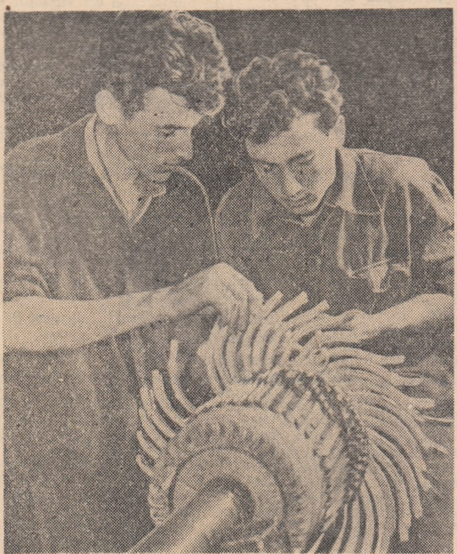
Iată, așa se execută corect operația de bobinare! Șteful Mihai, responsabilul unei brigăzi de producție a tineretului de la Uzina de motoare electrice București, îndrumă îndeaproape pe tinerii mai nou sosiți în brigadă.
