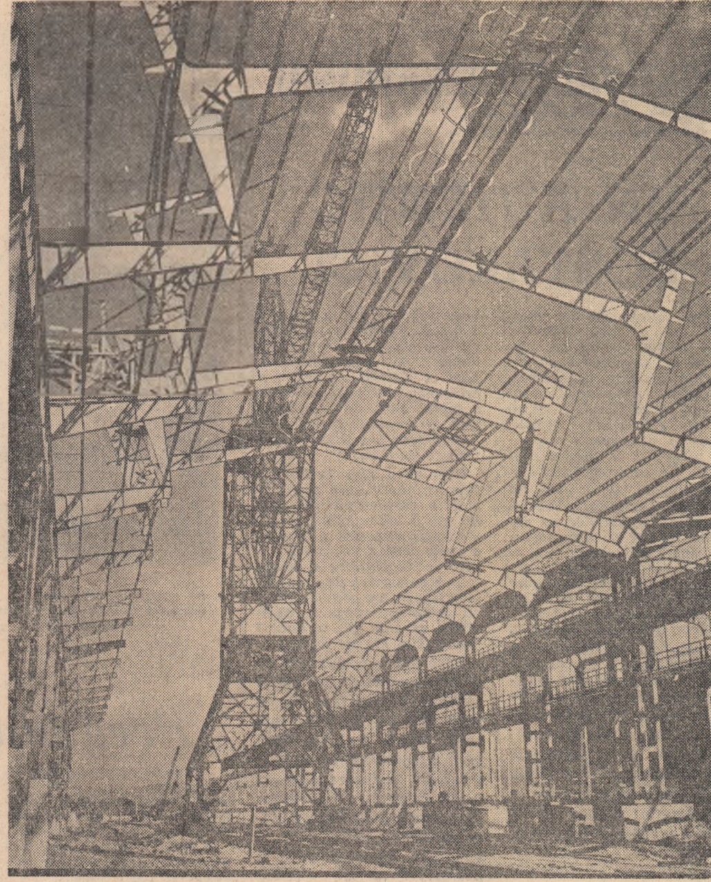
Artă și măiestrie. Muncitorii hunedoreni construiesc o linie de profile mijlocii pentru noul laminor.
