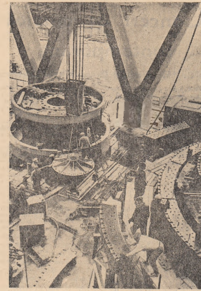
Un aspect de pe șantierele uriașe hidrocentrale de la Bratsk în curs de construire. În fotografia pe care o reproducem mai sus se lucrează la fundația viitoarei clădiri hidrocentralei
