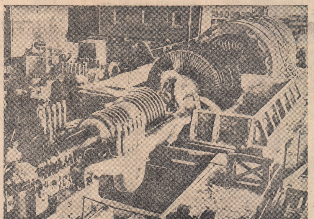
Lucrările de montare a celui de-al doilea turbogenerator de la centrala electrică de la Nazarov (U.R.S.S.).
