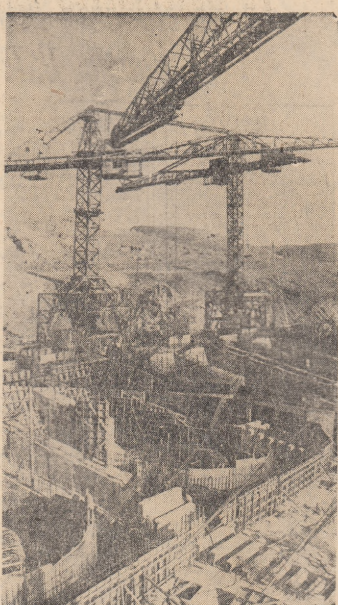
Hydrocentrala GOLOVNA (R.S.S. TADJICA) în curs de construire
