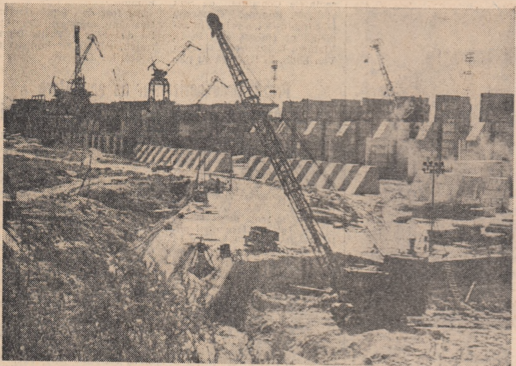
U.R.S.S.: Pe șantierul centralei hidroelectrice Dneproderjinsk. Constructorii și-au luat angajamentul ca pînă în ziua deschiderii Congresului al XXI-lea al P.C.U.S. să toarne 600.000 metri cubi de beton și să termine montarea stațiilor hidroagregate. În foto: vedere de ansamblu a șantierului de construcție.
