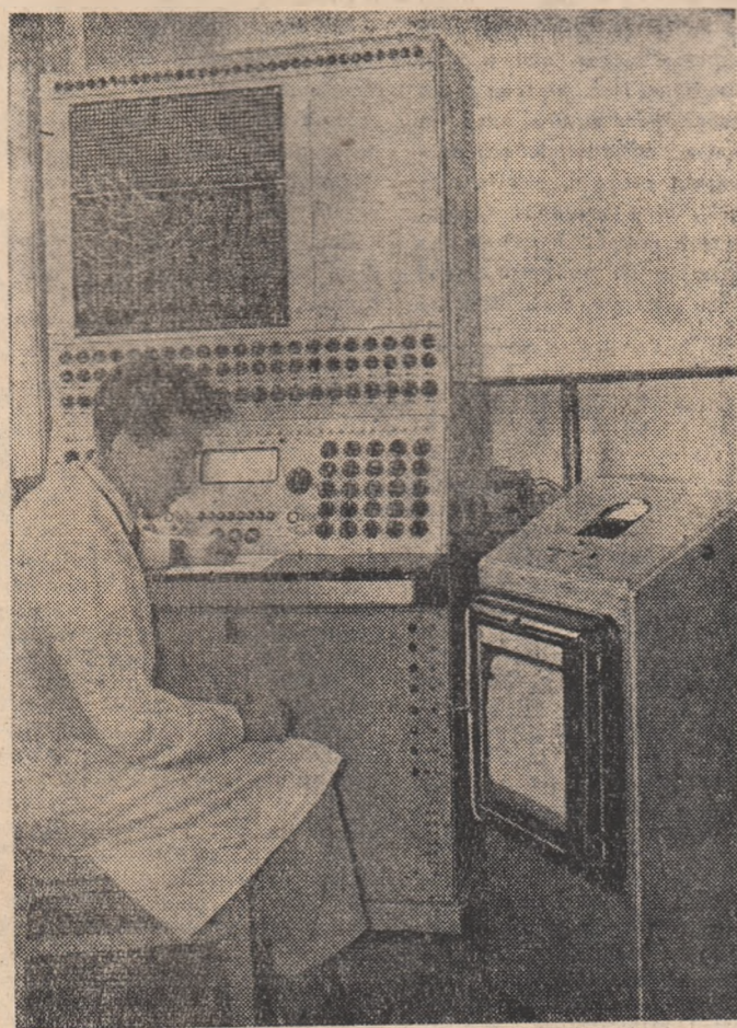
Mașina de calcul analogică pentru studiul reactorilor nucleari. În fotografia: inginerii Popu, Coșeni, unul dintre realizatorii mașinii urmărind funcționarea ei.
