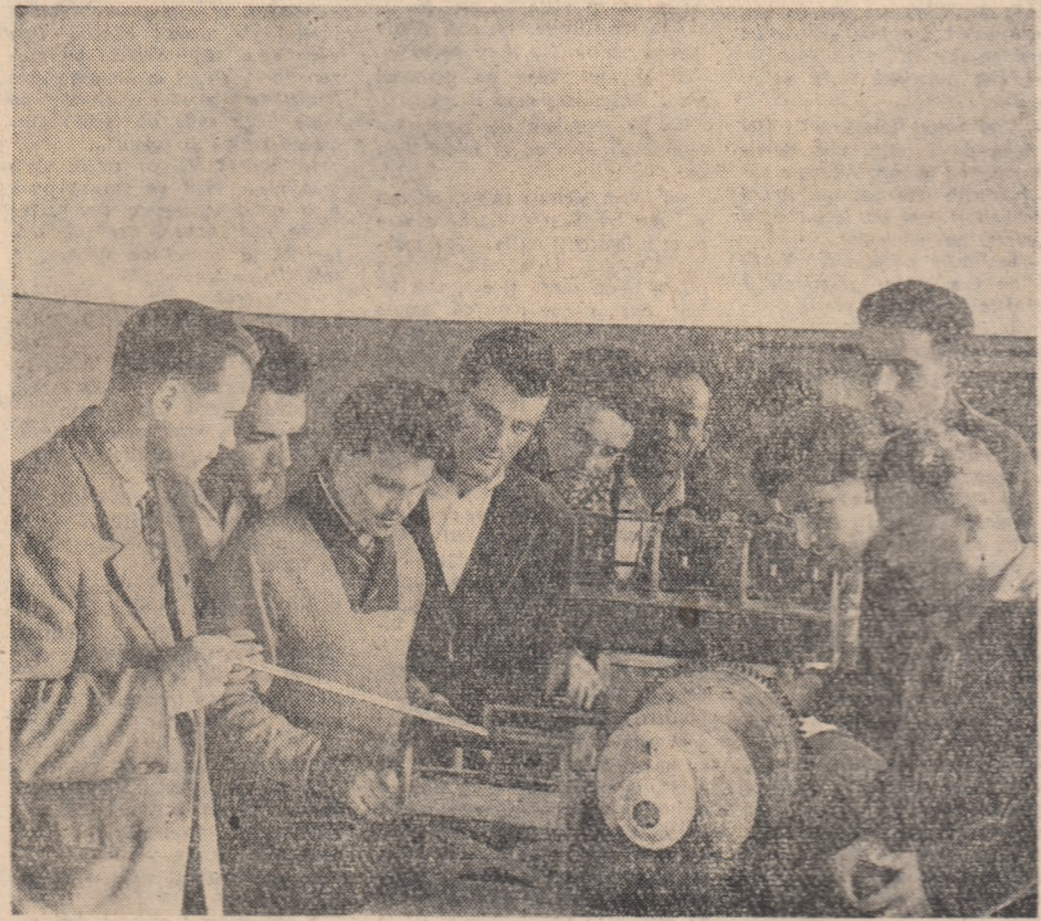
Instalația electrică a tractorului este foarte mult supusă solicitărilor. De aceea tinerii Nicolae Nistor și Vasile Cepoi de la Uzinele de tractoare din Brașov realizează cu maximum de atenție fiecare conexiune.
