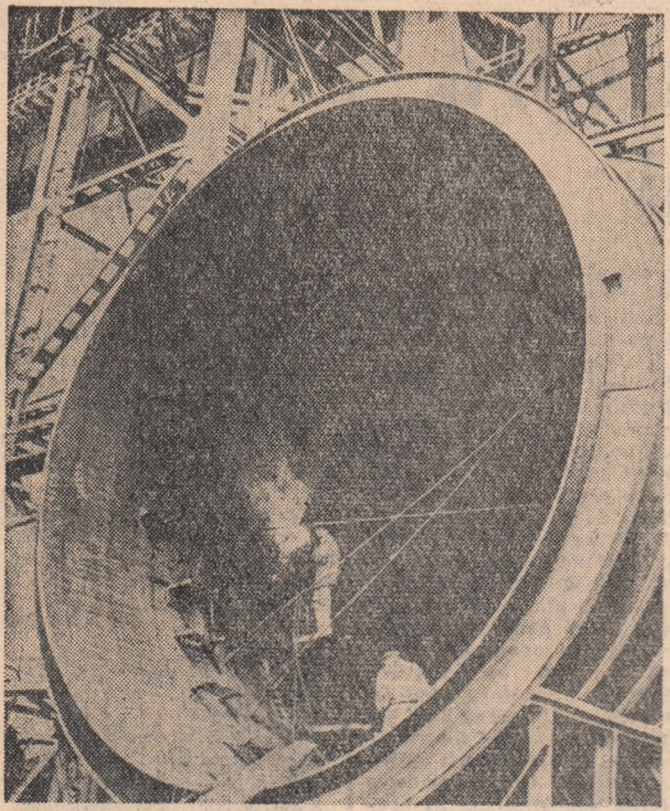
Aspect de pe șantiierul hidrocentralei de la BRATSK; executarea lucrărilor de sudură la conducta de apă a hidrocentralei
