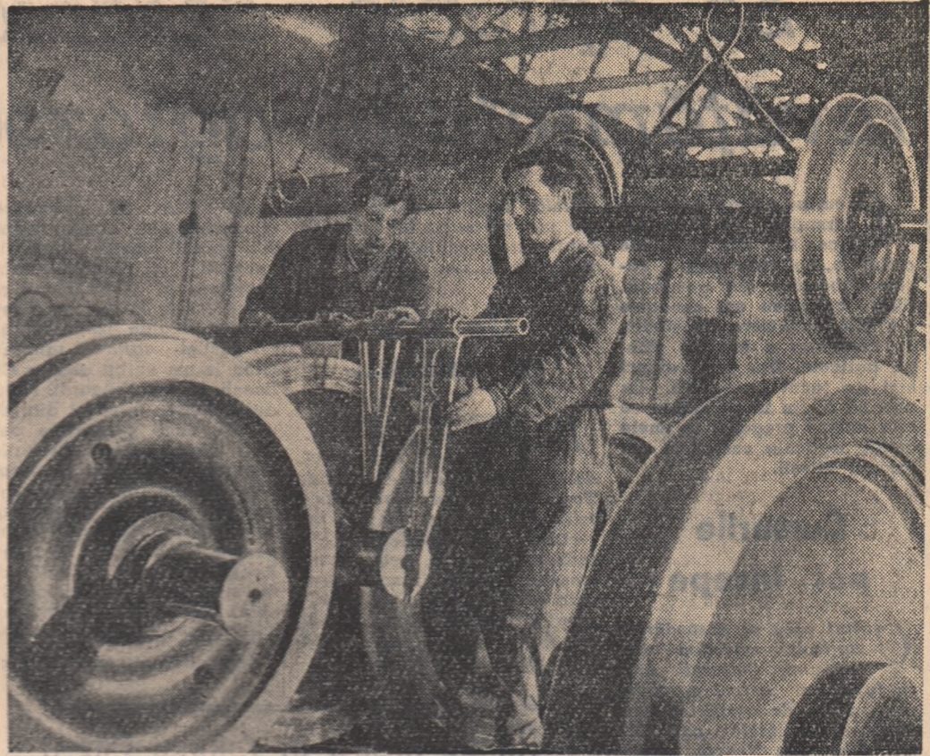
În secția rotării vagoanelor a Uzinelor „Ghișia roșie” din Capitală. Constantin Popa, responsabil de brigadă, împreună cu rotatorul Gh. Ionăiță măsoară simetria roților de vagoane înainte ca ele să plece spre hala de montaj.
