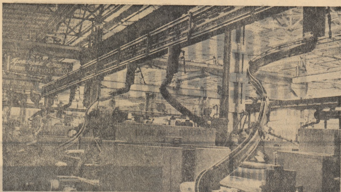
Cea de-a doua secție automată pentru producerea de rulmenți speciali la Uzina de rulmenți din Moscova.
