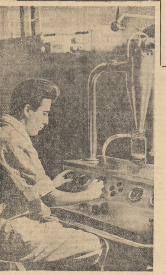
În laboratorul secției de industrie a lăptelui de la Institutul de Cercetări alimentare, se stabilește și se elaborează cu ajutorul liniei experimentale, tehnologia de fabricare a diferitelor produse lactate.
