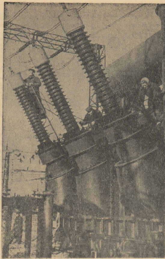
U.R.S.S.: Montarea unui transformator la termocentrala Zmievska-Komsomolskaia lângă Harkov, unde va fi pus în funcțiune cel de-al II-lea bloc energetic de 200.000 KW
