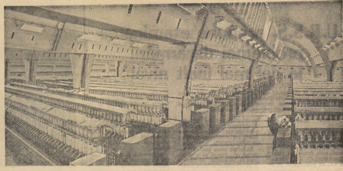
Mașini noi, moderne, luminate fluorescent. Așa și-a spus cuvîntul tehnica modernă în secția șinguri din noua filatură de la Găvana-Pitești
