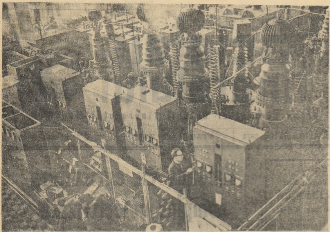
Noua aparatură experimentală a laboratorului de redresori de înaltă tensiune al Institutului unional electrotehnic „V. I. Lenin” din Moscova.
