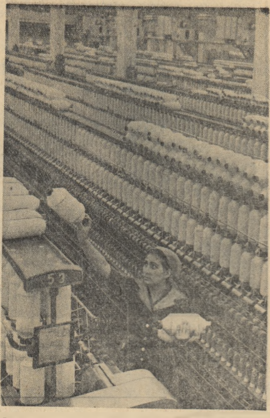
Aspect din secția ring de la Bumbăcăria Jilava din Capitala. Foto: AGERPRES
