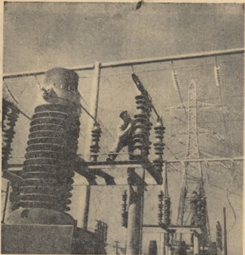
Stieja de transformare a energiei electrice Titan din Capitală se dezvoltă prin instalarea unor noi transformatori. Lucrările le execută muncitorii întreprinderii de construcții și montaje energetice București. În fotografie: Se montează separatorii de 110 Kv. Foto: AGERPRES
