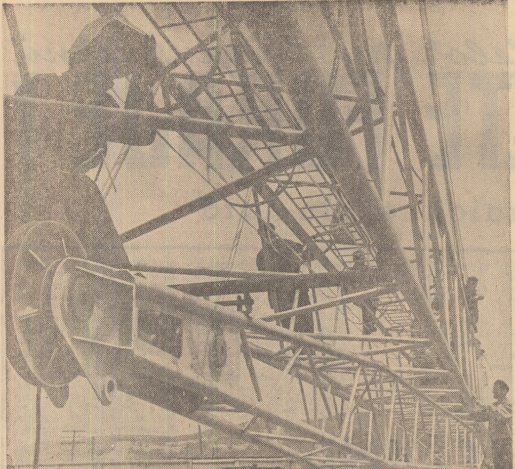
Pentru construcțiile de locuințe și șantierul industrial din țara noastră, la Uzinele de construcții metalice și mașini agricole din Bocșa, regiunea Banat, a intrat în fabricație un nou lot de macarale turn de 40 T.m.
