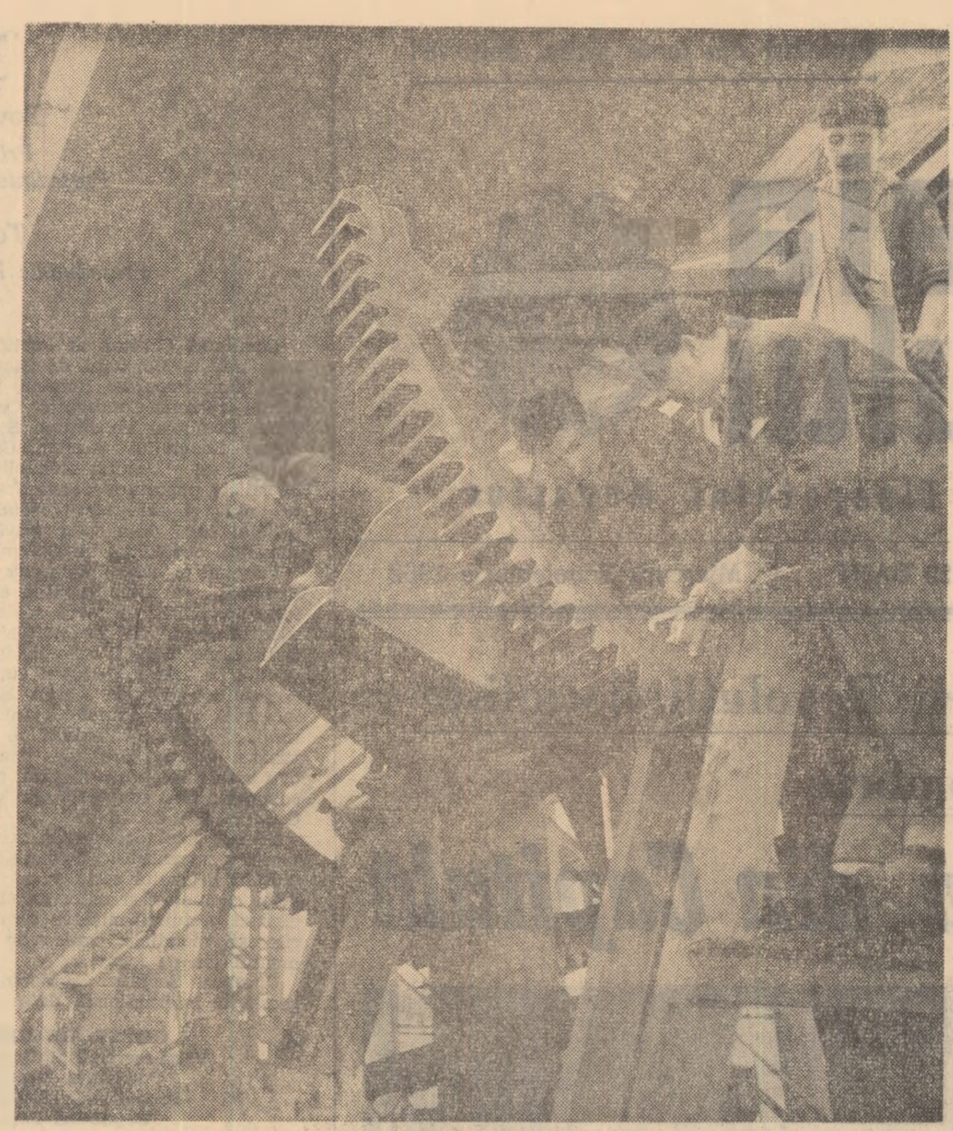
Uzinele „23 August” din Capitală. Alături de muncitorii vîrstnici din brigada condusă de Ilie Feher, din secția construcții mecanice, tinerii Viorel Cristescu, Oprea Gh. și Moșog Marin lucrează la montarea mecanismelor unor mașini grele necesare industriei siderurgice.
