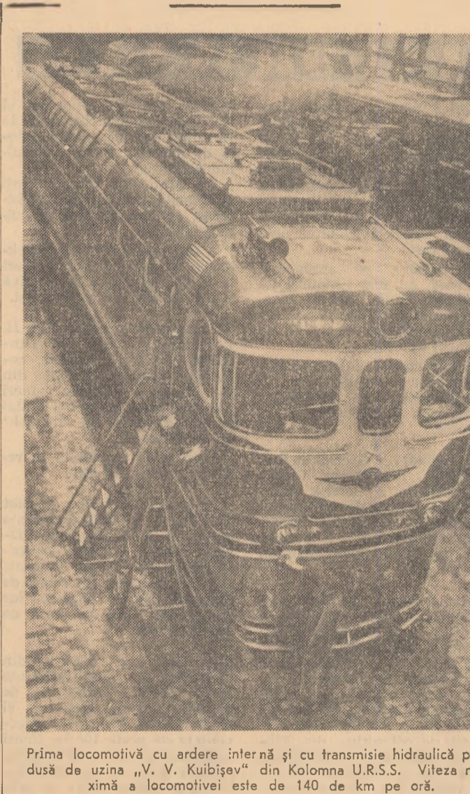
Prima locomotivă cu ardere internă și cu transmisie hidraulică produsă de uzina „V. V. Kubișev” din Kolomna U.R.S.S. Viteza maximă a locomotivei este de 140 de km pe oră.
