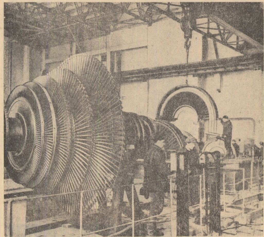
Montarea principalei turbine de aburi a centralei atomoelectrice I. V. Kurchatov din apropiere de Sverdlovsk.
