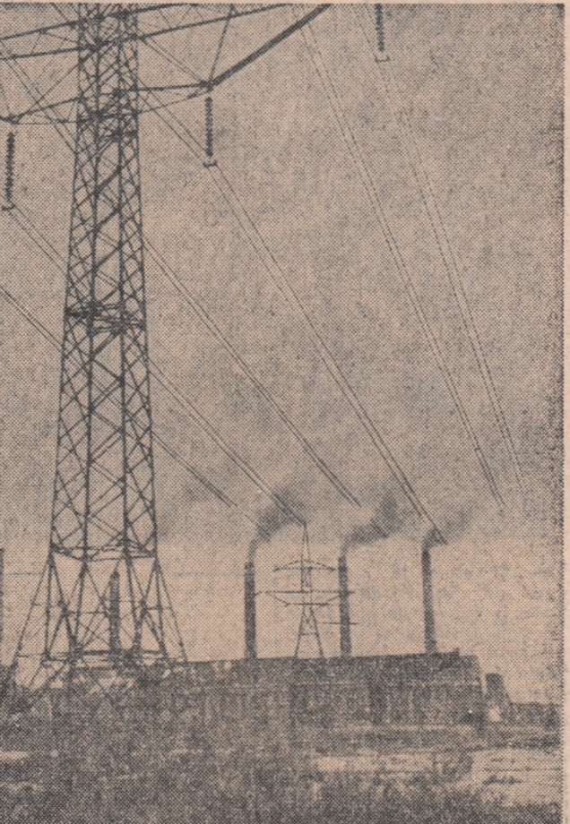
La uzinele termocentrale sovietice, printre care și la cea din Uralul de sud, au fost instalate turbine și generatoare cu o capacitate de 200.000 kW. În fotografie: aspect exterior al termocentralei din Uralul de sud.
