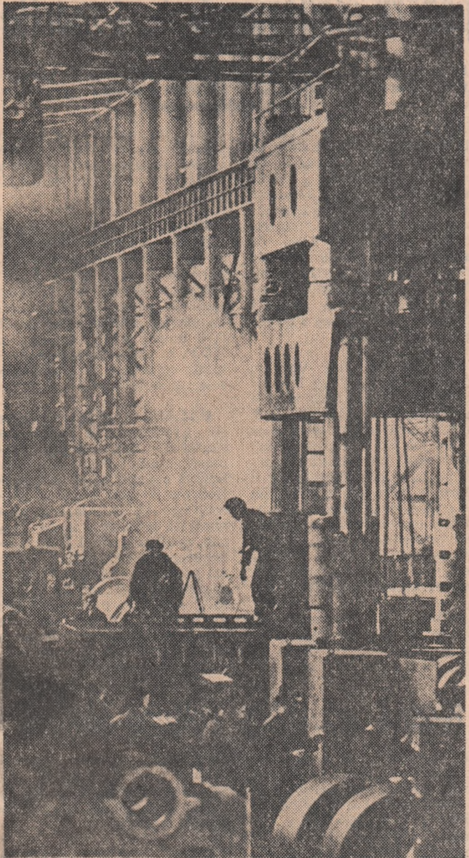
Noua presă hidraulică verticală cu o putere de 3150 tone instalată recent la uzina de strunguri din Kolomen (U.R.S.S.).
