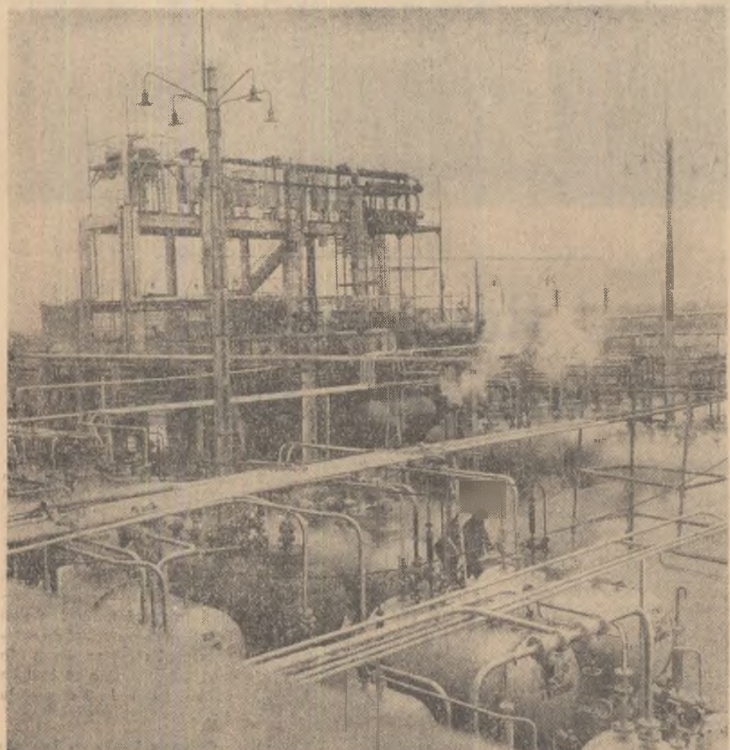
Vedere generală a instalației pentru rectificarea și recuperarea alcoolilor și izonitrizare din cadul secției de sinteză a fabricii de medicamente „Terapia” din Cluj. Foto: AGERPRES
