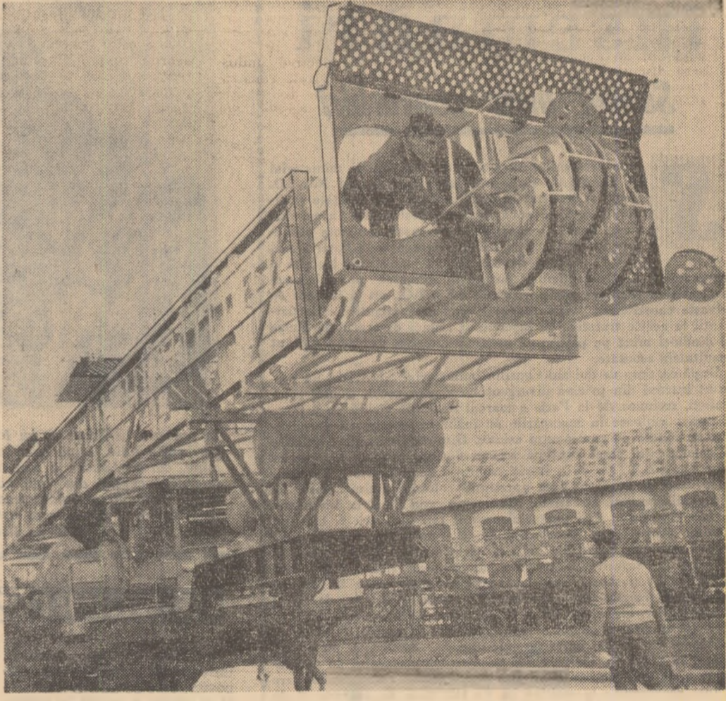
Un grup de muncitori de la Uzinele „I. Mai”-Ploiești, execută ultimele lucrări de verificare a instalației de toraj T. 50, care lăcătează pînă la 1200 metri adîncime. Foto: AGERPRES
