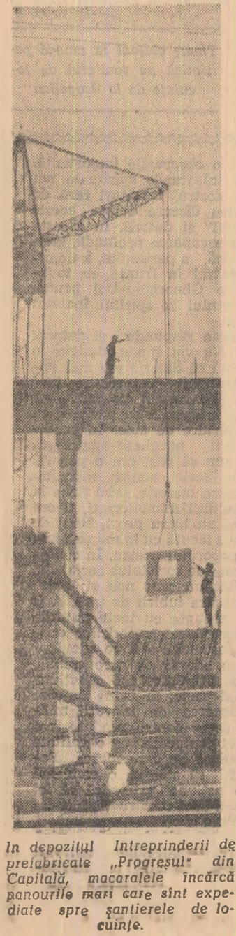
În depozitul întreprinderii de prelucrare „Progresul” din Capitală, macaralele încarcă panourile mari care sint expediate spre șantieretele de locuințe.
