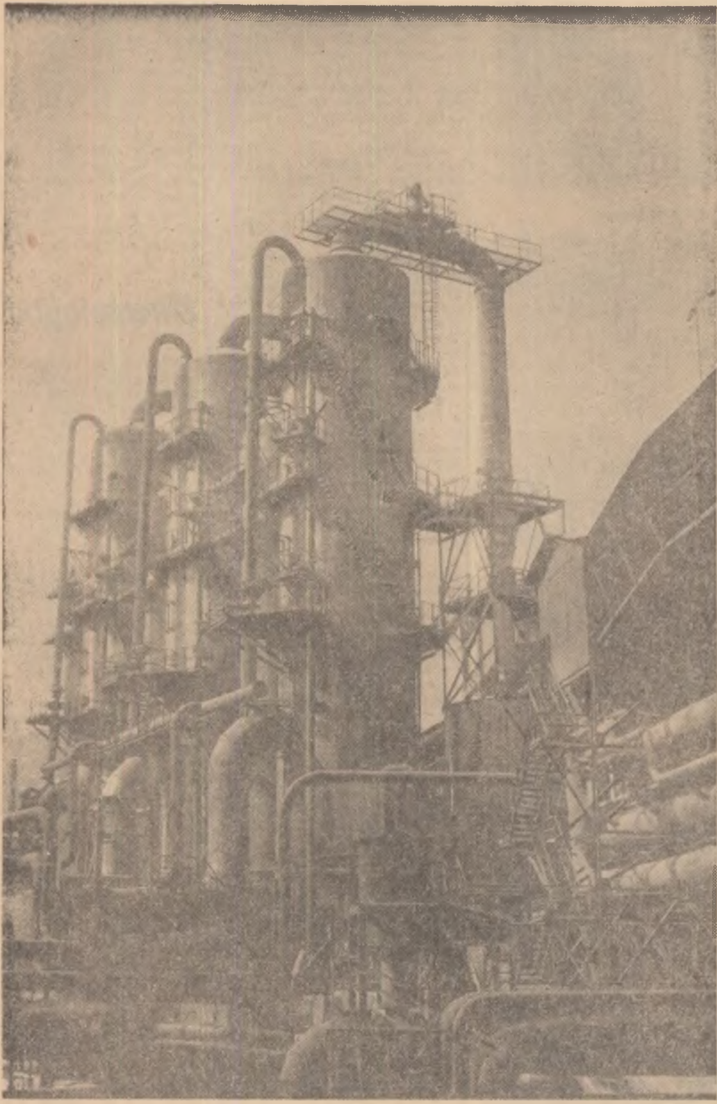
Instalația de încălzire a aerului de la furnalul de 700 mc al Combinatului siderurgic Reșița. Foto: AGERPRES
