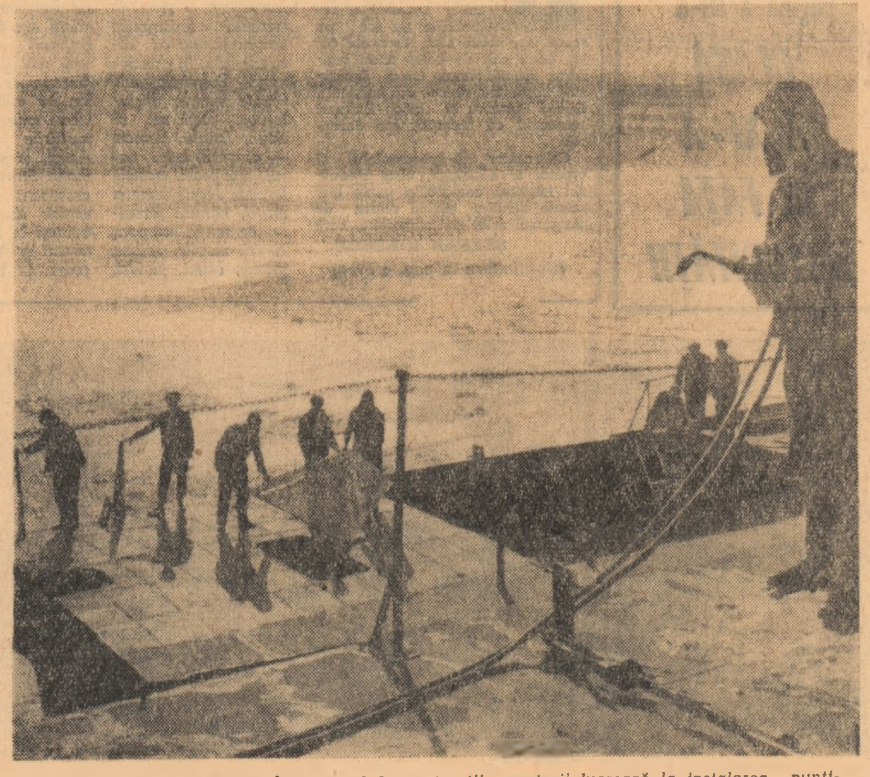
Șantierul Naval Otlenița. În sectorul I construcții, montorii lucrează la instalarea punții — partea centrală și pupa — unei motonave de 2000 tone. Foto: AGERPRES
