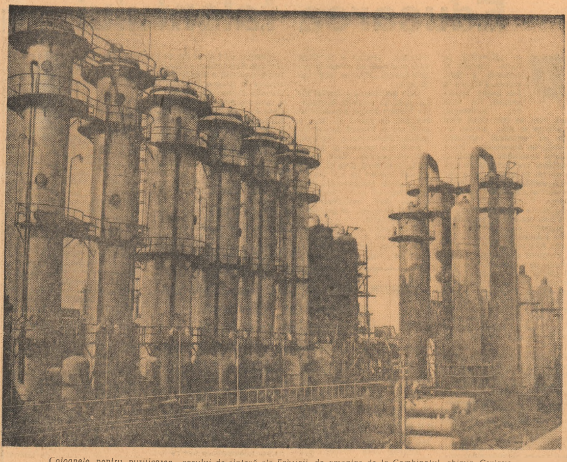
Coloanele pentru purificarea gazului de sinteză ale Fabricii de amoniac de la Combinatul chimic Cruiova. Foto: AGERPRES
