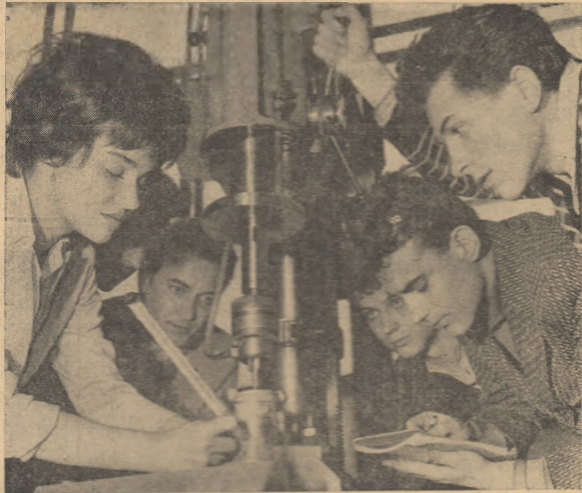
Studentii anului III de la Facultatea de mecanică a Institutului politehnic Timișoara determină cantitatea de căldură deșchisă în procesul de așchiere a metalelor în laboratorul de mașini unelte.
