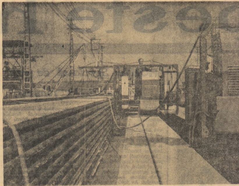
La Intreprinderea de prefabricate „Progresul” din Capitală, tăierea fișilor cu goluri din beton precomprinat se execută cu utilaje de mare randament
