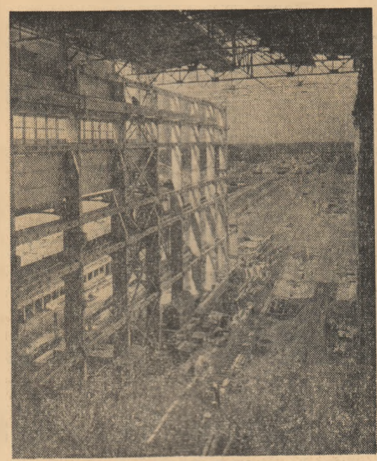
U.R.S.S.: Aspect de pe sanctorul centralei electrice de la Konakovo. Foto: A.P.N.
