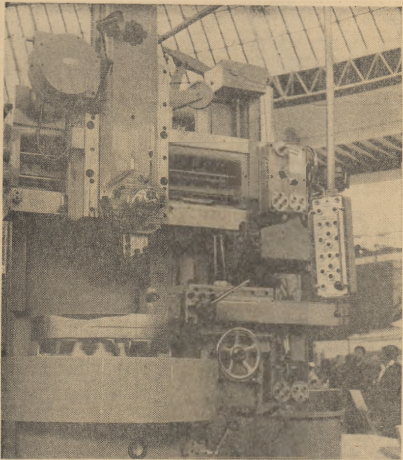
Strungul Carusel — SC-2.500 produs de Fabrica de mașini unelte și agregate-București care poate prelucra piese cu un diametru de 2.700 mm și înălțimea de 1.900 mm având greutatea de 15 tone.
