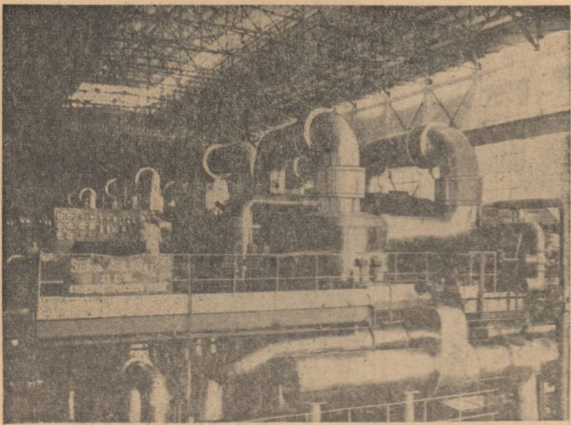
U.R.S.S.: Vedere generală a sălii mașinilor de la Centrala atomo-electrică din Voronej.
