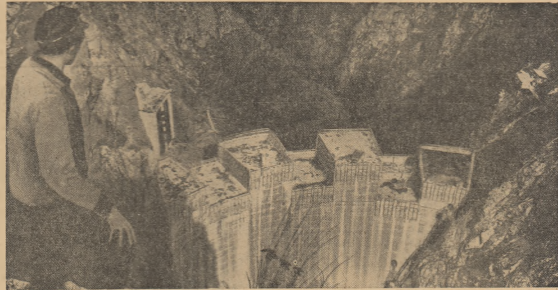
Construcții de pe șantierul barajului hidrocentral „16 Februarie” de pe Argeș au ridicat barajul pînă în prezent la o înălțime de peste 70 m. În fotografie — imagine de pe șantier Foto: AGERPRES
