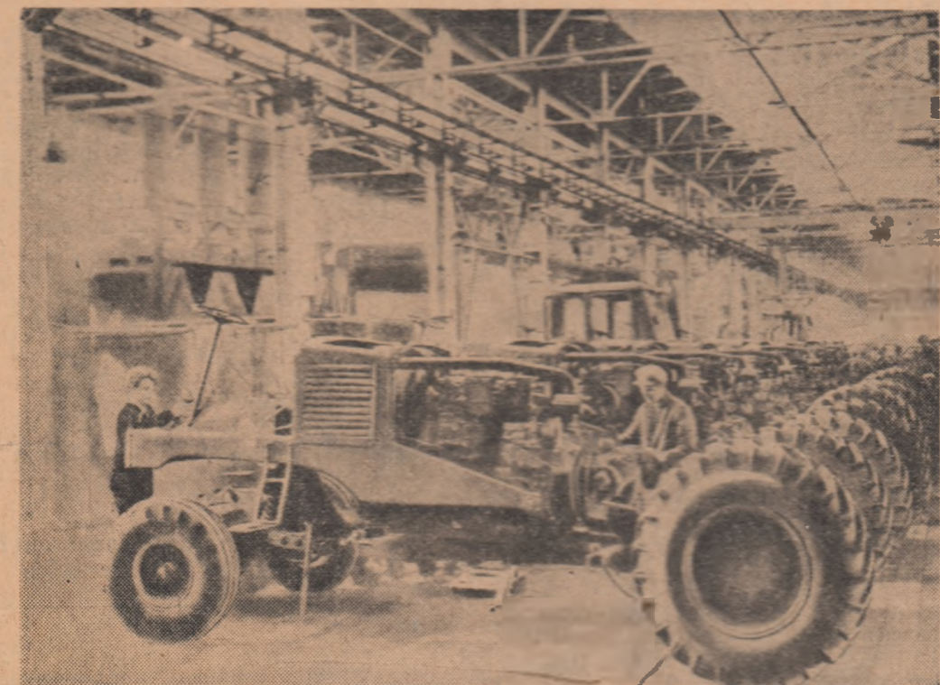
U.R.S.S. Asamblarea unui lot experimental de sașuri universale la o uzină din Taganrog
