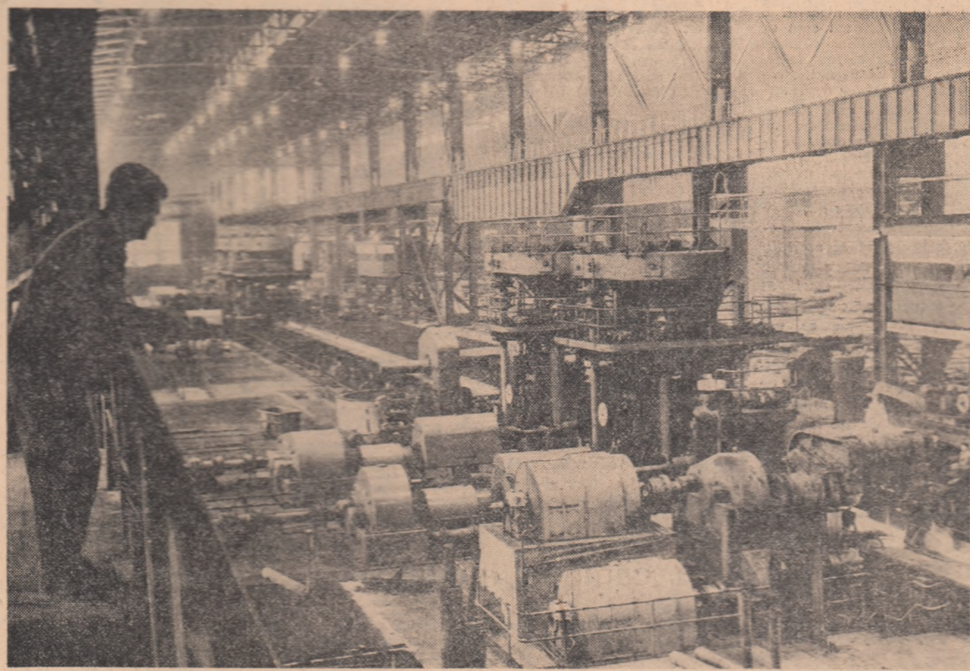
Laminorul continuu de semilabricate de la Combinatul siderurgic Hunedoara
