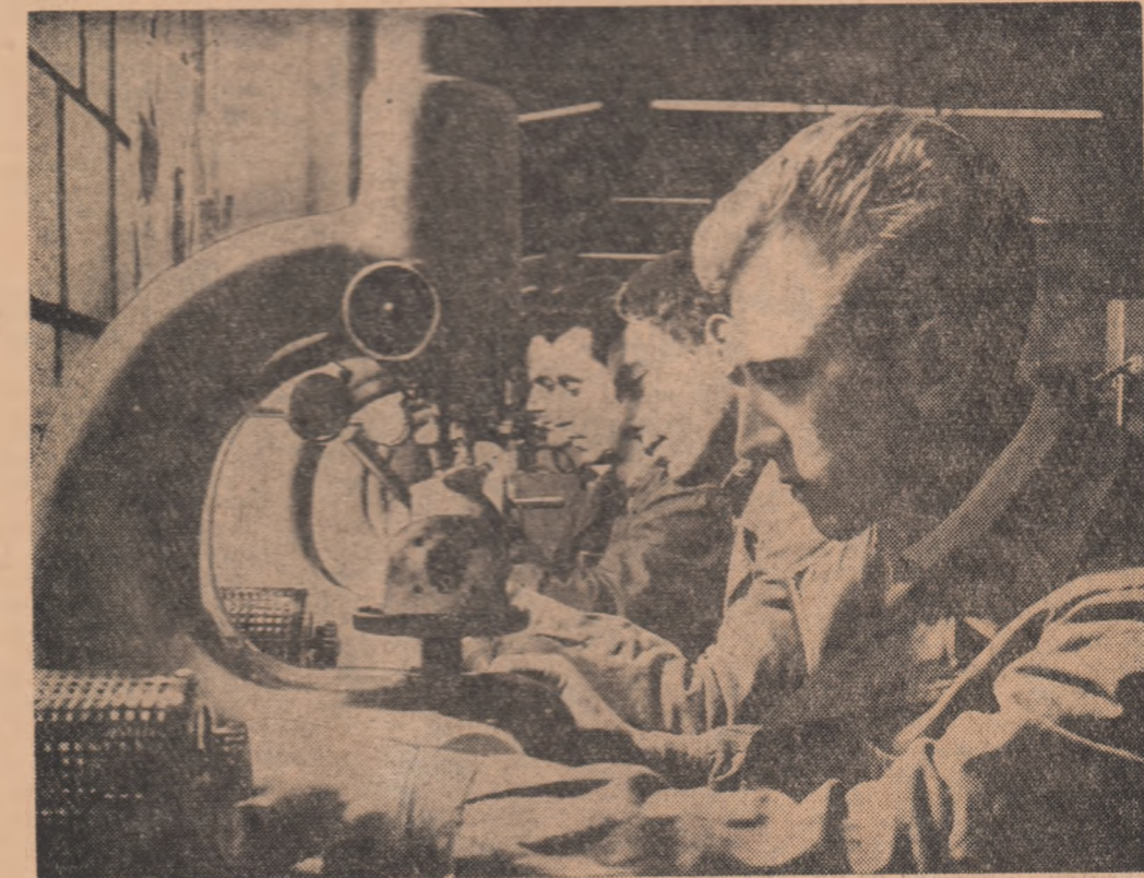
Tinerii de la Uzina mecanică-Sinai, datorită pregătirii lor profesionale, minulesc cu pricepere mașini dintre cele mai moderne. Ită-i în prim plan, pe Gh. Olaru și Ion Rosca lucrînd la o mașină de rectificat pulverizatoare, care are 16 000 de ture pe minut
