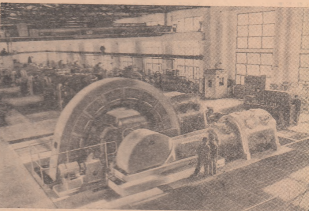
R. P. CHINEZĂ: Compresorul de nitrogen, intrat recent în funcțiune la Fabrica chimică experimentală din Pekin
