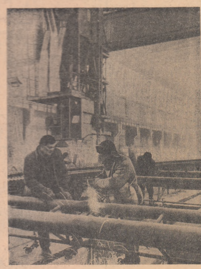
La Uzina de aluminiu Slatina se montează poduri rulante la secția de electroliză (fotografia din stînga). Și iată de asemenea (sus) lucrîndu-se la montarea scheletului metalic al injectoarelor secției cuptoare-coa cere
