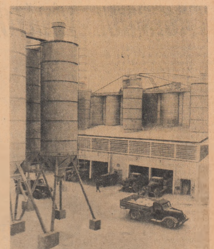
În cartierul Balta Albă, în apropiere de noile construcții ce se ridică, funcționează stafia de preparare a betonului. A-cestă unitate de mare productivitate, dotată cu instalații moderne, produce în 24 ore betonul necesar pentru circa 70 de apartamente. În fotografie: vedere a stației de preparare a betonului Foto: AGERPRES
